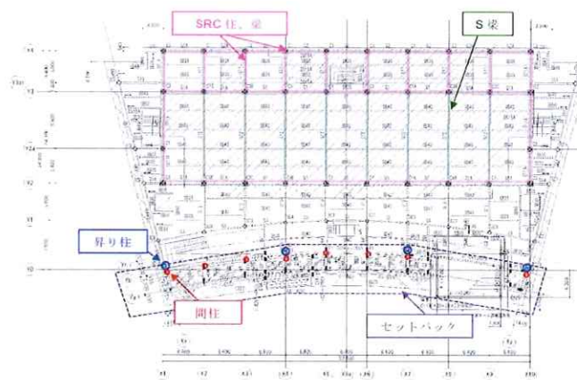
【新庁舎棟】構造架構伏図
