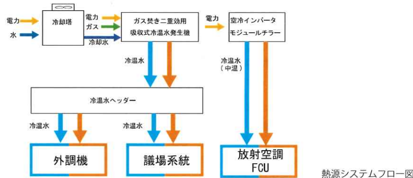
熱源システムフロー図
