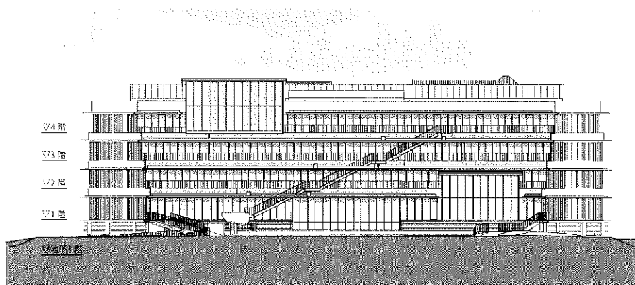
◇南立面図
