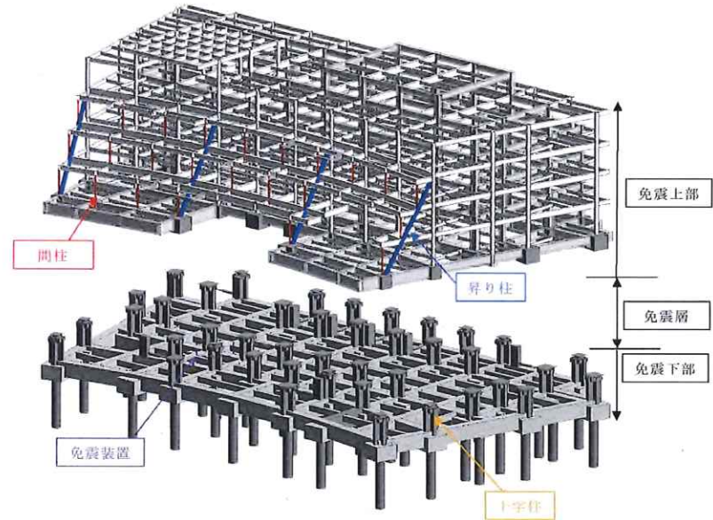
【新庁舎棟】構造架構パース
