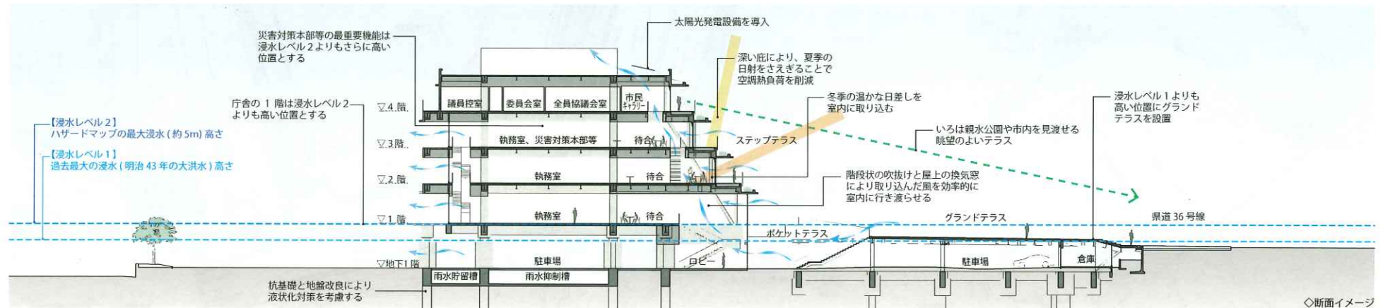
◇断面イメージ
