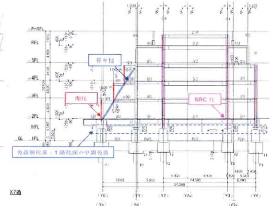
【新庁舎棟】構造架構軸組図
